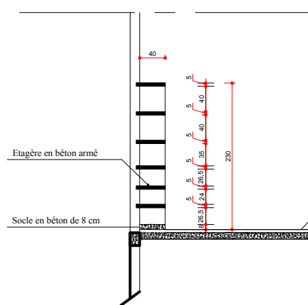
COUPE SUR BIBLIOTHEQUE
