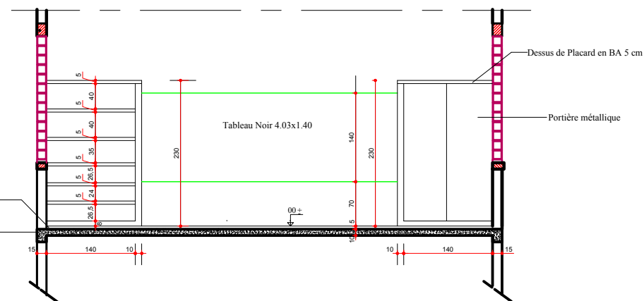
BIBLIOTHEQUE ET PLACARD VUE EN ELEVATION
