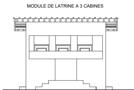
FACADE AVANT
